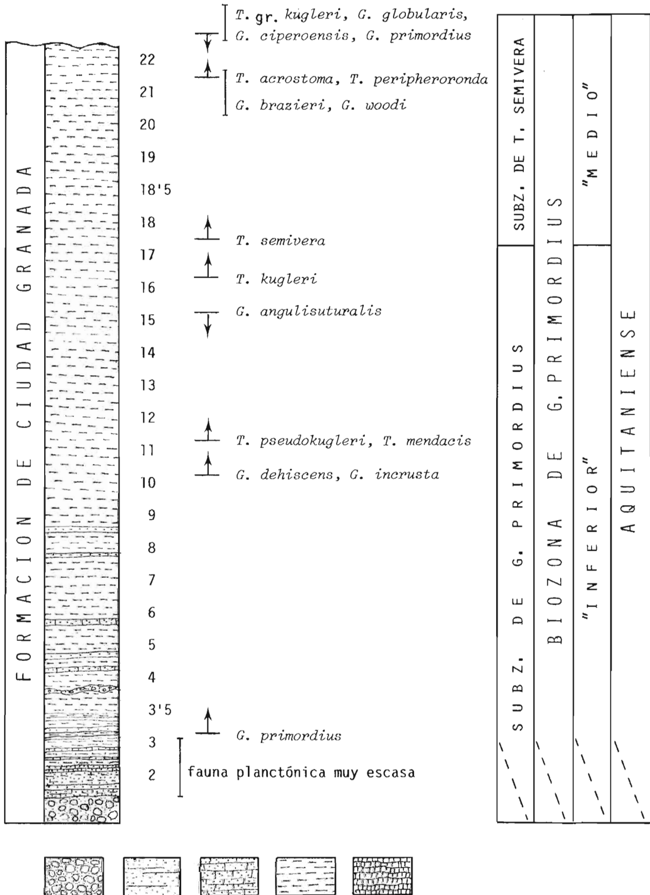
Fig. 2.—Formación de Ciudad Granada: Biohorizontes significativos, bioestratigrafía, cronoestratigrafía y esquema litológico (potencias relativas de los tramos no respetadas). 1: Conglomerados y brechas. 2: Arenas y areniscas. 3: Calcareenitas. 4: Arcillas y margas. 5: Silexites y tufitas.
